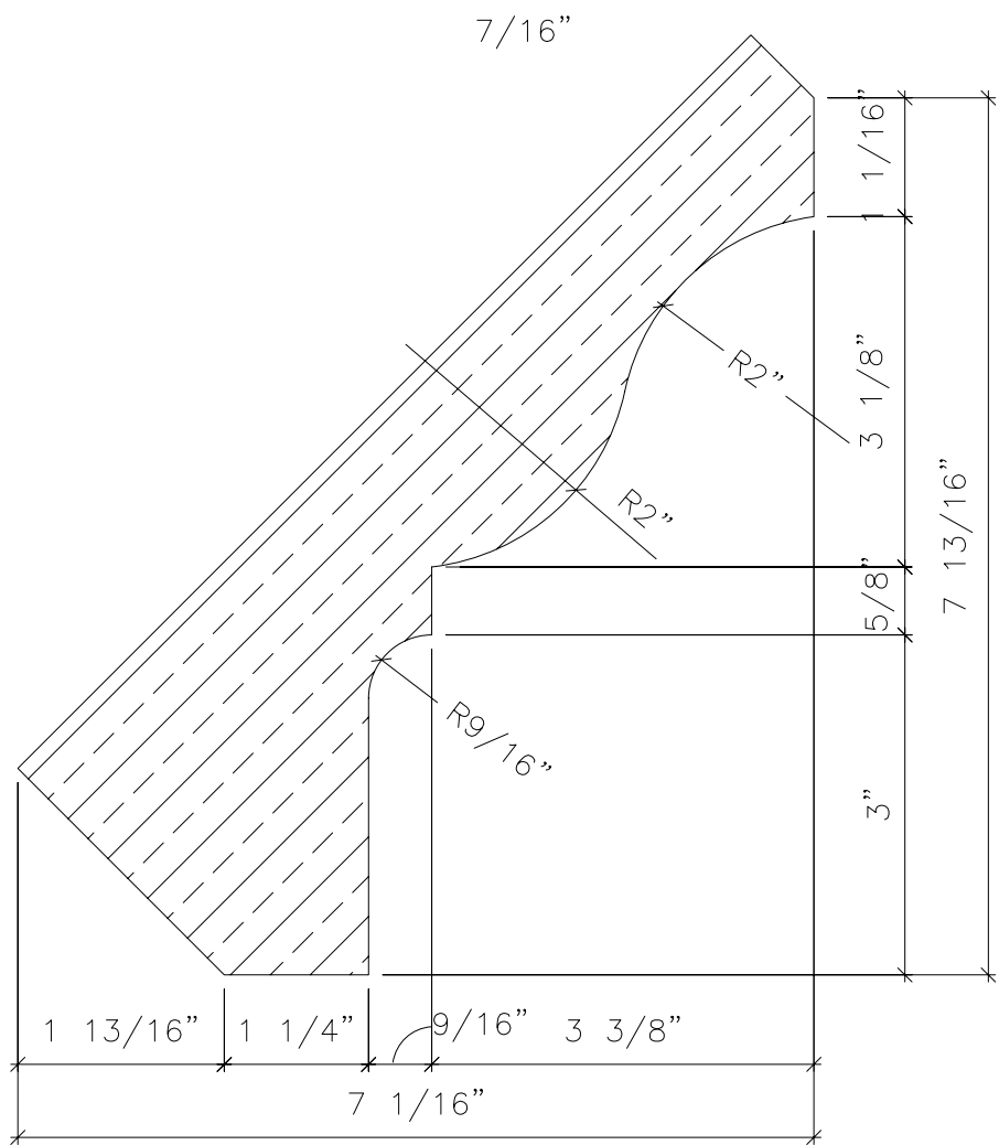
1 PROFILE 301-T
